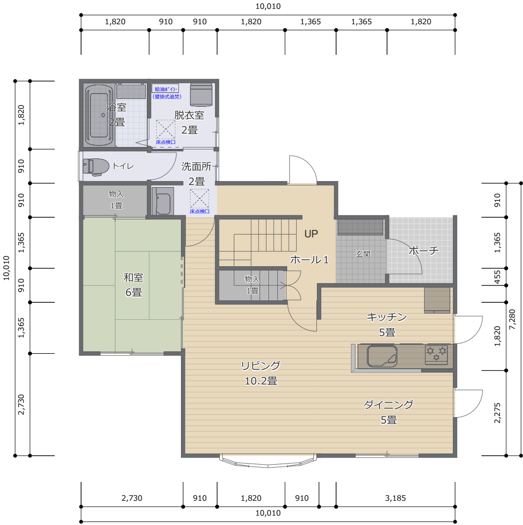
1階縮尺 1/100
